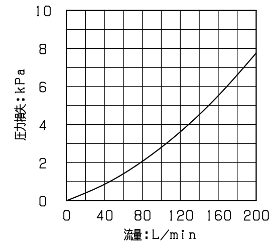
流量特性
